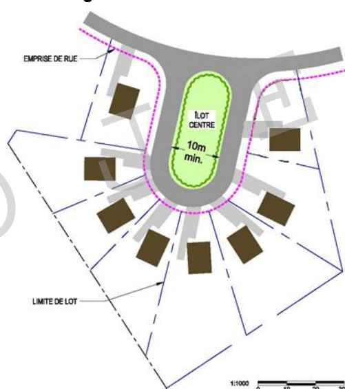
Figure 9.1 – Ilot résidentiel
