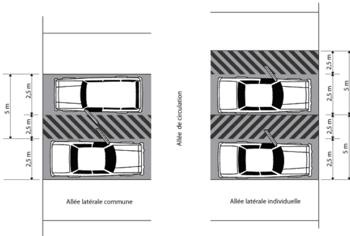
Figure 16 - Cases de stationnement réservées aux personnes handicapées avec allée latérale commune ou individuelle.
