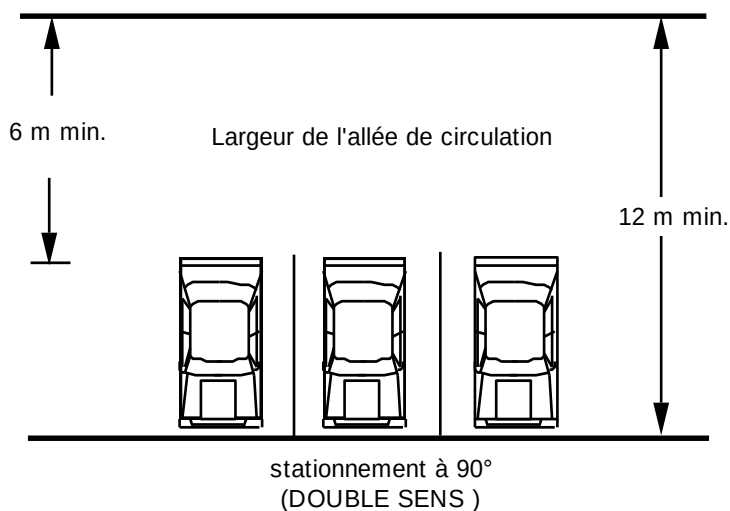
Figure 13 : Largeur d'une allée de circulation pour le stationnement à 90° à double sens
