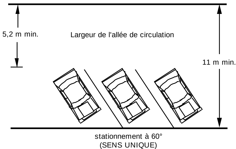
Figure 12 : Largeur d'une allée de circulation pour le stationnement à angle de 60° à sens unique
