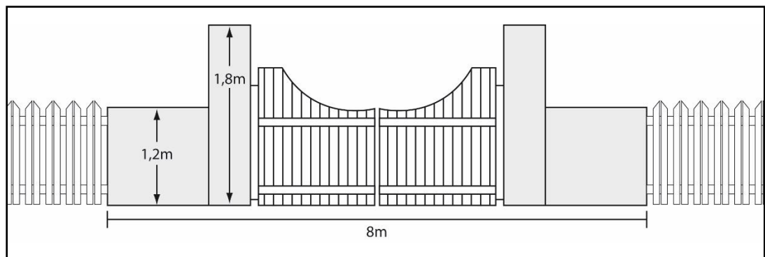
Figure 7 - Dimensions d'un portail d'entrée
