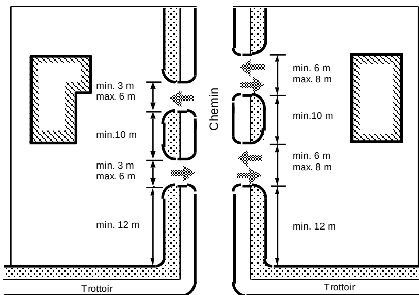
Figure 15 - Dimension des allées d'accès
