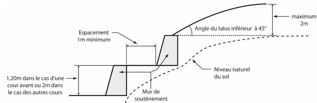
Figure 6 - Espace minimum requis entre deux murs de soutènement
