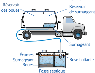
Étape 1 : Aspiration du surnageant contenu dans la fosse septique
