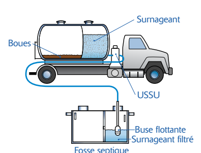
Étape 3 : Traitement du surnageant et retour à la fosse
